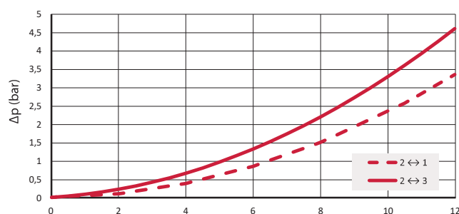
Perdite di carico/Pressure drop
